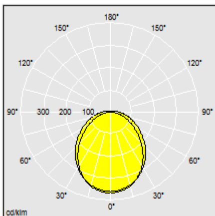
Curva Fotometrica
